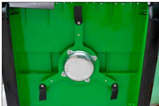
De BEV hakselaars zijn uitgerust met een rotor met 3 messen van het "TD type"
