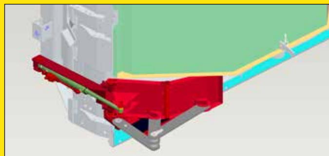
Strooikap met strooibegrenzingsluik(en)
