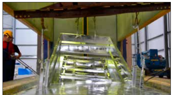
Thermisch verzinkingsbad (galvanisatie aan binnen- en buitenzijde)
